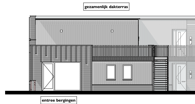
Kopgevel zuid
