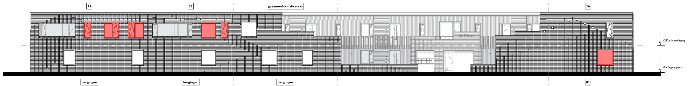
Westgevel
