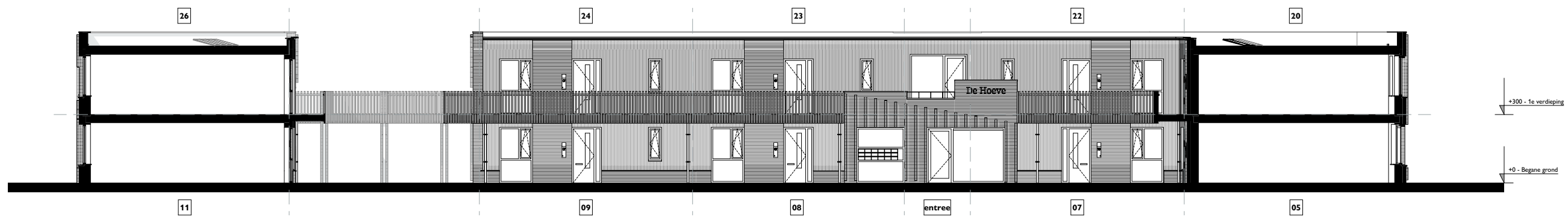
Westgevel binnen
