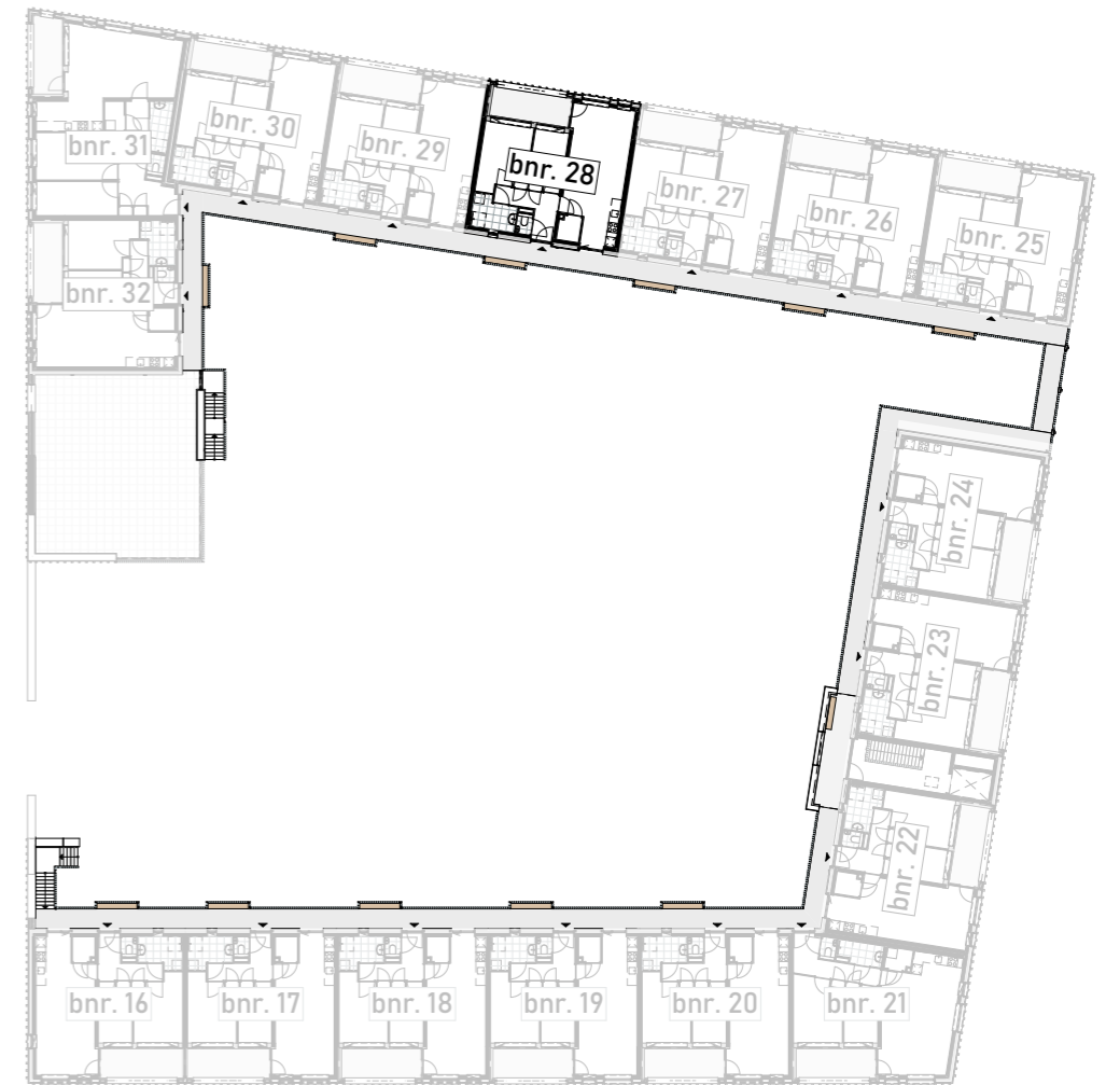
1e verdieping
