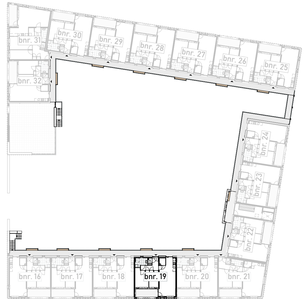
1e verdieping
